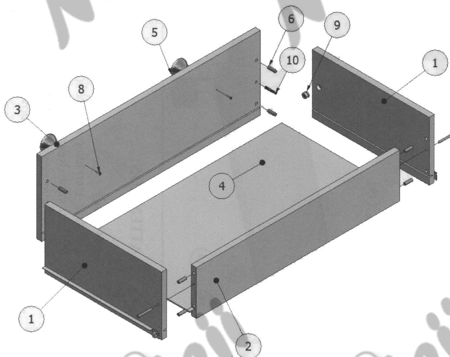
Vystimo lentos karkaso surinkimas
